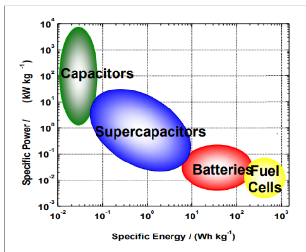
Figura 12: Ragone plot
